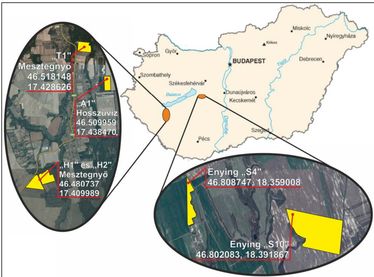
3.2. ábra. A kísérleti területek elhelyezkedése
