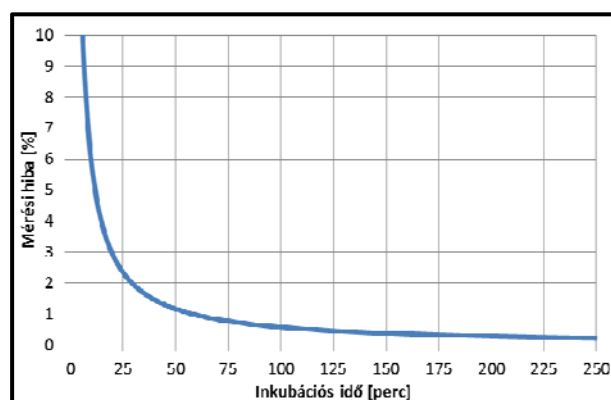
4.12. ábra. A mérési hiba az idő függvényében a mérőkamra 5 ppm koncentráció változása esetén
