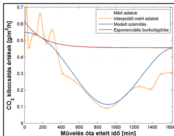
4.35. ábra. A kibocsátási modell illeszkedése a 10. mérés tárcsázott területen mért adataira
