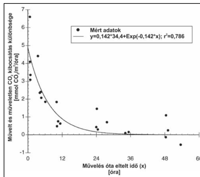
2.15. ábra. A talajművelés utáni CO 2 kibocsátás és közelítése exponenciális függvényvel Forrás: (ELLERT és JANZEN, 1999)
