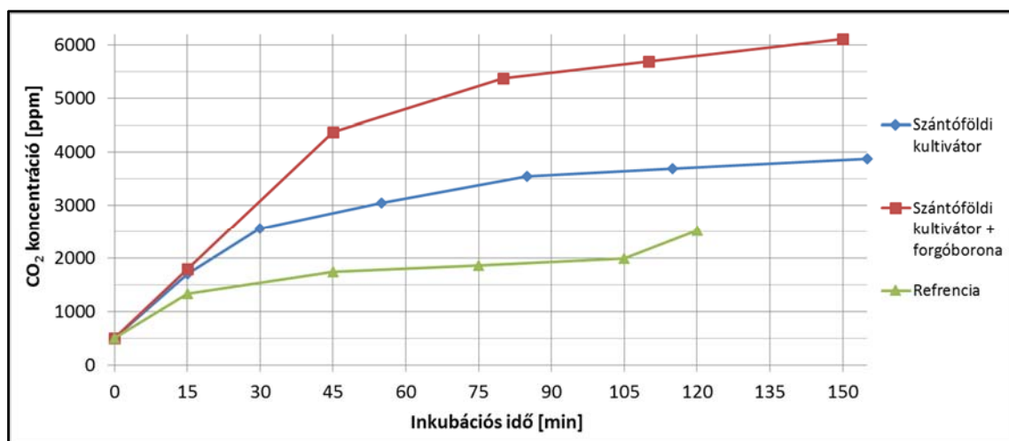
4.5. ábra. A mérőkamrák CO 2 koncentrációjának változása az inkubációs idő függvényében (4. mérés)
