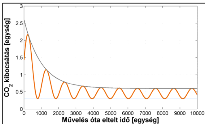
4.26. ábra. A (4.7) egyenlet grafikus megoldásának jellegábrázolása
