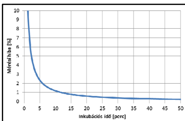
4.11. ábra. A mérési hiba az idő függvényében a mérőkamra 1 ppm koncentráció változása esetén
