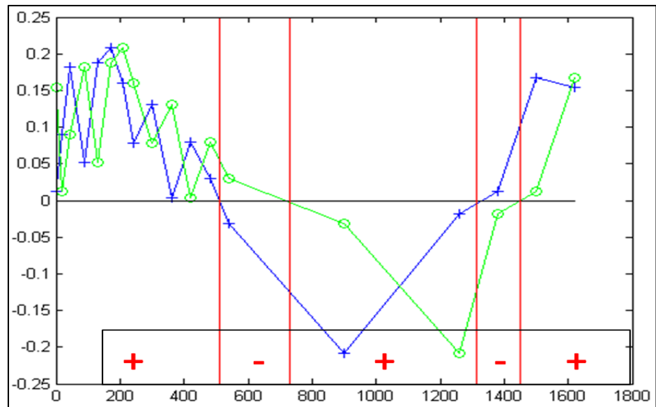
4.27. ábra. A mért adatok periódusidejének meghatározásához szükséges eredeti és egy hellyel léptetett függvényértékek szorzatának előjelvizsgálata
