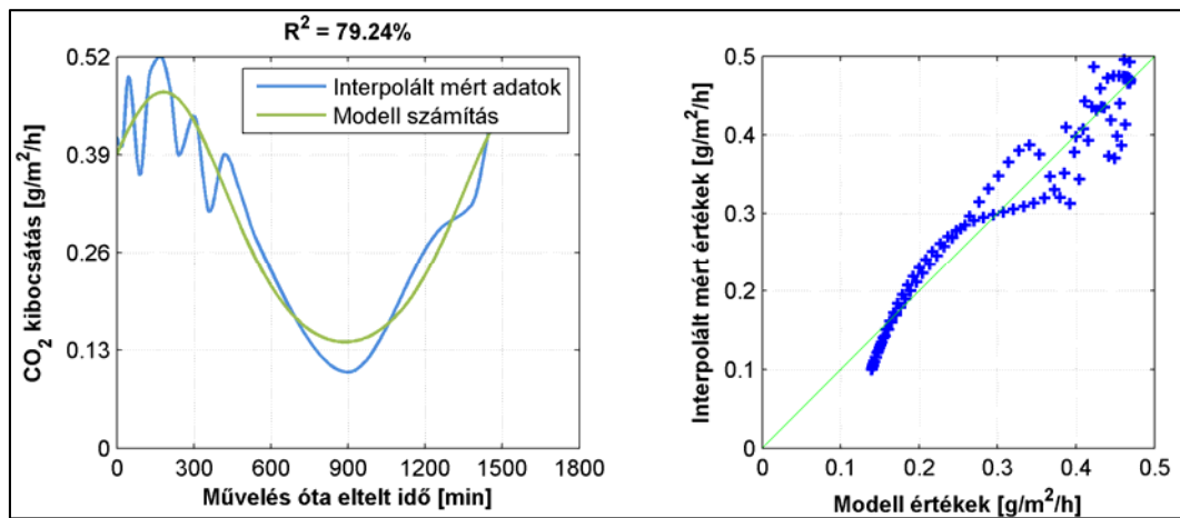
4.38. ábra. A kibocsátási modell O'Connell modellel kiegészített szinuszos tagjának illeszkedése a műveletlen terület interpolált mért adataira (10. mérés)
