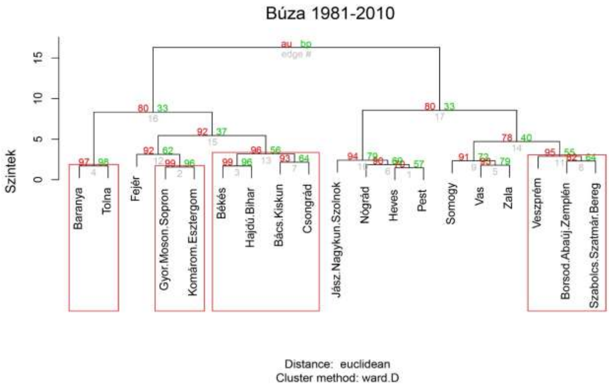
4f ábra Az 1981–2010 közötti megyei búza termésátlagok hierarchikus klaszterei. AU = közelítő bizonytalanságot tükröző p-érték, BP = bootstrap valószínűség p-értéke. Vörös keretben azok a klaszterek szerepelnek, amelyekben AU \geq 95 .
