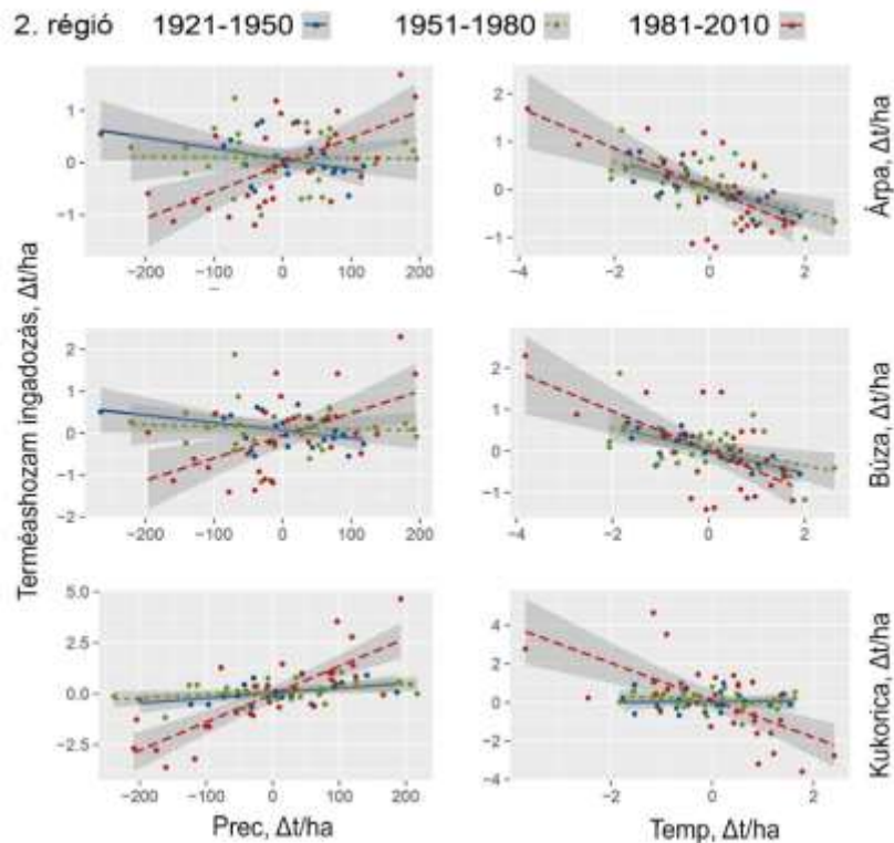
9b ábra Klimatikus változók és a 2. régió (Észak-Dunántúl) termésátlagainak első differencia értékei közötti kapcsolatok szórásgörbéi 30 éves periódusokban (1922–2010). A sötétszürke sávok a determinisztikus kapcsolatok 95%-os konfidencia intervallumát mutatják. Prec = vegetációs időszakos csapadékösszegek, Temp = vegetációs időszakos hőmérsékleti átlagok.
