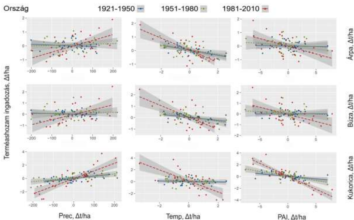
8. ábra Klimatikus változók és az országos termésátlagok első differencia értékei közötti kapcsolatok szórásgörbéi 30 éves periódusokban (1921–2010). A sötétszürke sávok a determinisztikus kapcsolatok 95%-os konfidencia intervallumát mutatják. Prec = vegetációs időszaki csapadékösszegek, Temp = vegetációs időszaki hőmérsékleti átlagok, PAI = a Pálfai féle aszályindex országos átlagai.
