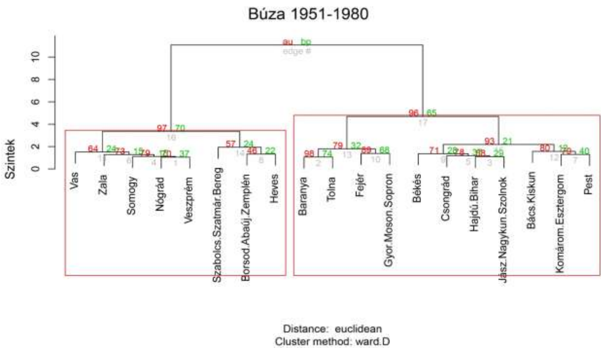
4e ábra Az 1951–1980 közötti megyei búza termésátlagok hierarchikus klaszterei. AU = közelítő bizonytalanságot tükröző p-érték, BP = bootstrap valószínűség p-értéke. Vörös keretben azok a klaszterek szerepelnek, amelyekben AU \geq 95 .
