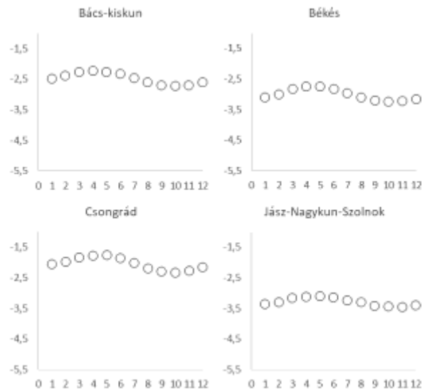
7e ábra A talajvízmélység havi átlagainak alakulása az 5. gabonatermesztési régió megyéiben (1981–2010)
