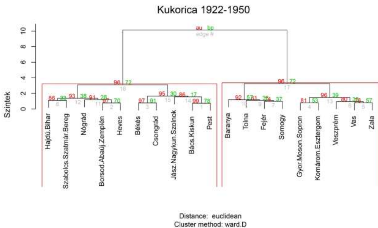
4g ábra Az 1922–1950 közötti megyei kukorica termésátlagok hierarchikus klaszterei. AU = közelítő bizonytalanságot tükröző p-érték, BP = bootstrap valószínűség p-értéke. Vörös keretben azok a klaszterek szerepelnek, amelyekben AU \geq 95 .
