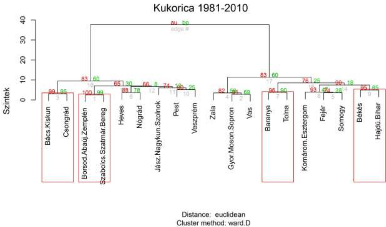
4i ábra Az 1981–2010 közötti megyei kukorica termésátlagok hierarchikus klaszterei. AU = közelítő bizonytalanságot tükröző p-érték, BP = bootstrap valószínűség p-értéke. Vörös keretben azok a klaszterek szerepelnek, amelyekben AU \geq 95 .
