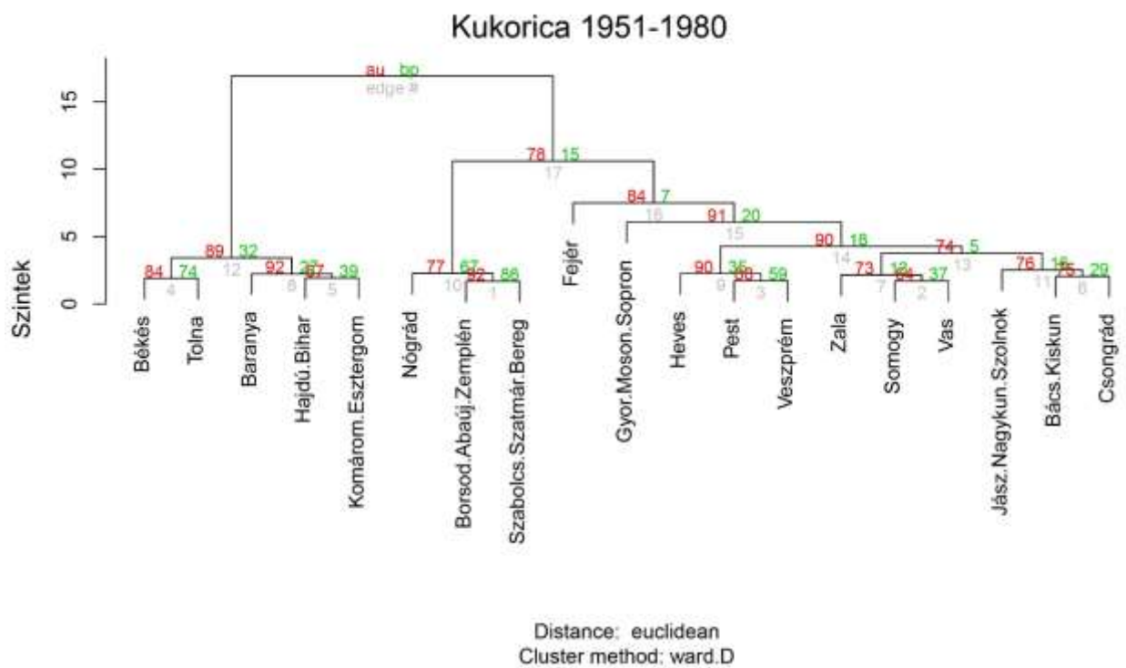
4h ábra Az 1951–1980 közötti megyei kukorica termésátlagok hierarchikus klaszterei. AU = közelítő bizonytalanságot tükröző p-érték, BP = bootstrap valószínűség p-értéke. Vörös keretben azok a klaszterek szerepelnek, amelyekben AU \geq 95 .
