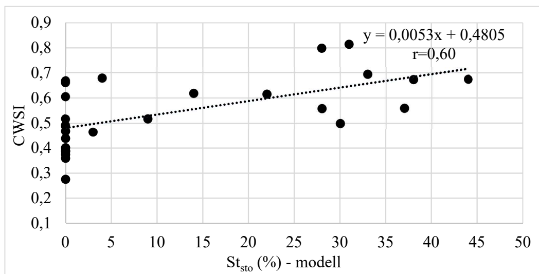
70. ábra: A modellezett vízstressz ( St_{sto} %) és a méréseken alapuló értékek (CWSI) kapcsolata 2017. júliusában a kontrollban ( n=27 ).
